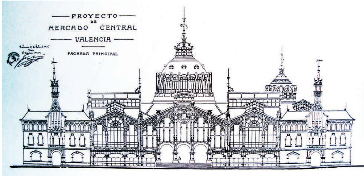
Alçat de conjunt: façana de l'entrada principal i pavellons administratius (1915).
