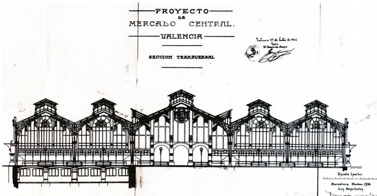
Secció trasversal del Mercat Central i detall de soterranis.
